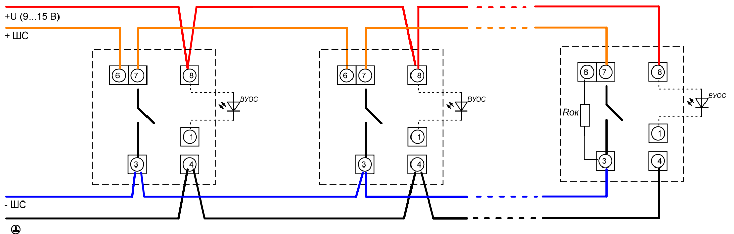
рис.3 "Подключение ИП 212-xxx с UC-02. Вар.3
