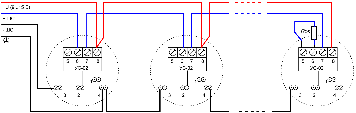
рис.1 "Подключение ИП 212-xxx с UC-02. Вар.1
