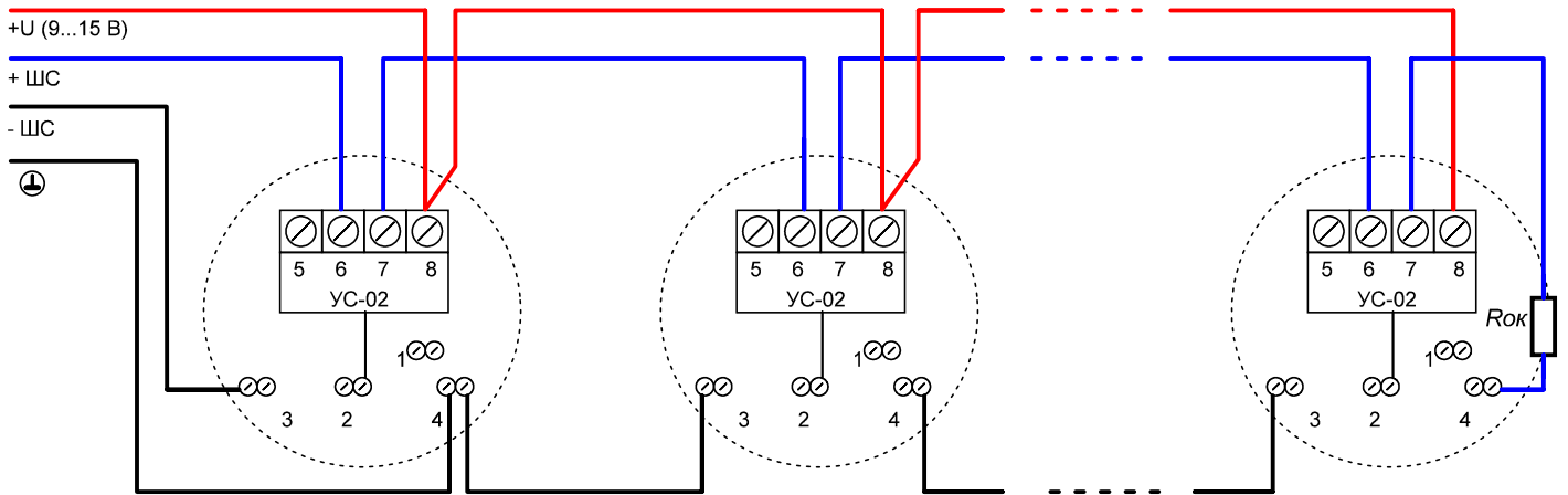
рис.2 "Подключение ИП 212-xxx с UC-02. Вар.2
